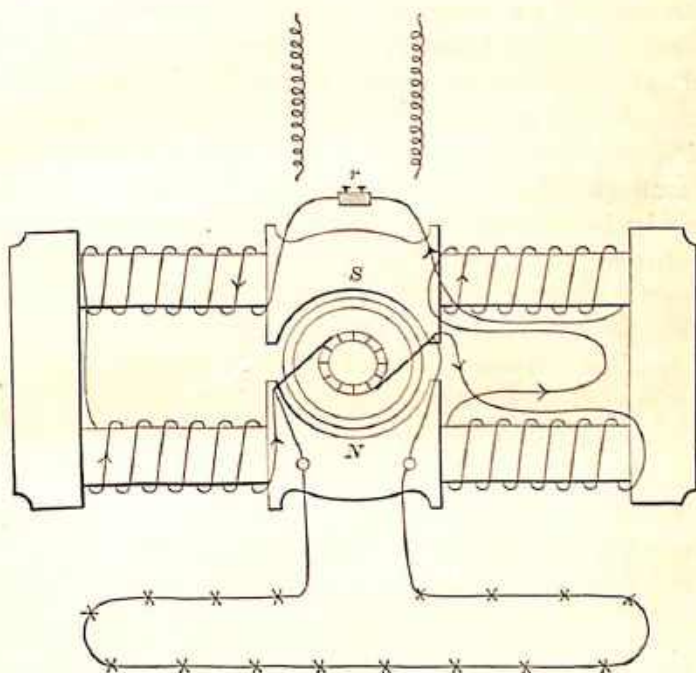
Fig. 6.—Shunt Wound Dynamo.
