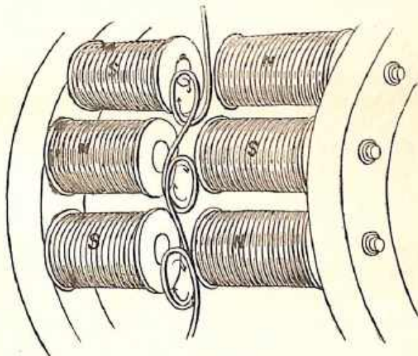
Fig. 9.—Siemens Machine.
